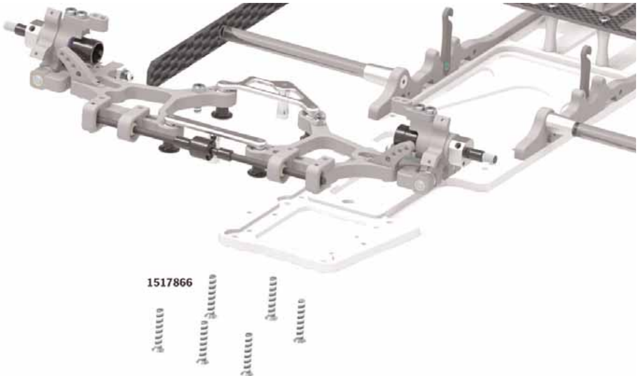
Querlenker hinten oben und Getriebeplatte/A-arm rear upper and transmission bracket
